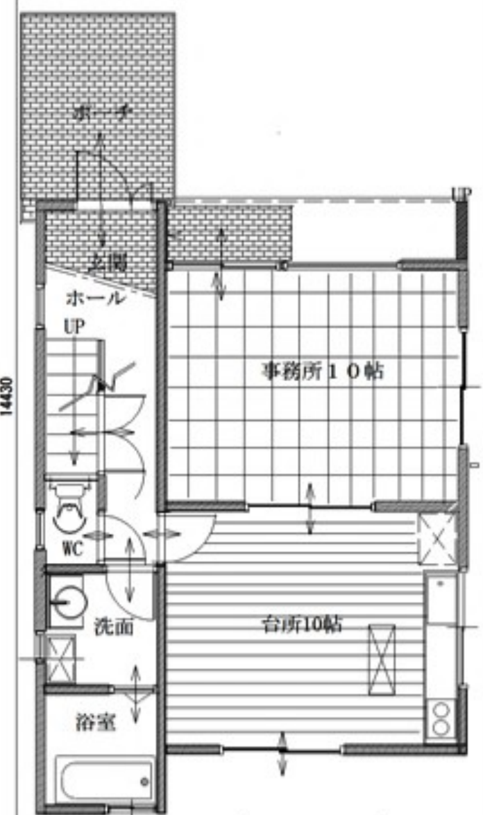
1階平面図
