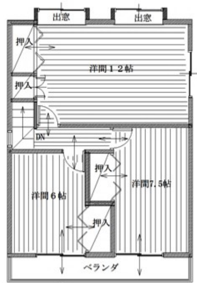
3階平面図
