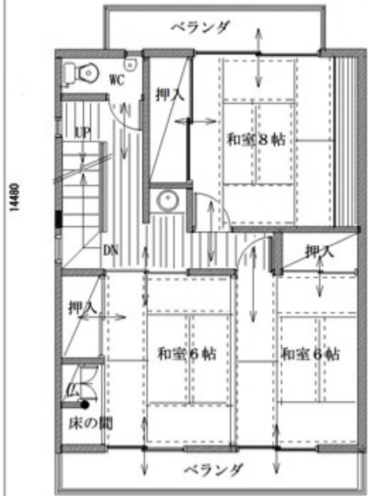
2階平面図
